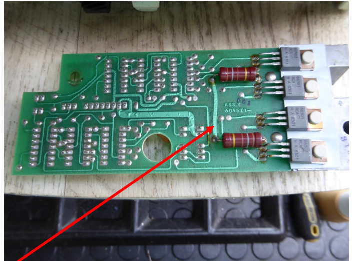
Obere Steuerplatine
