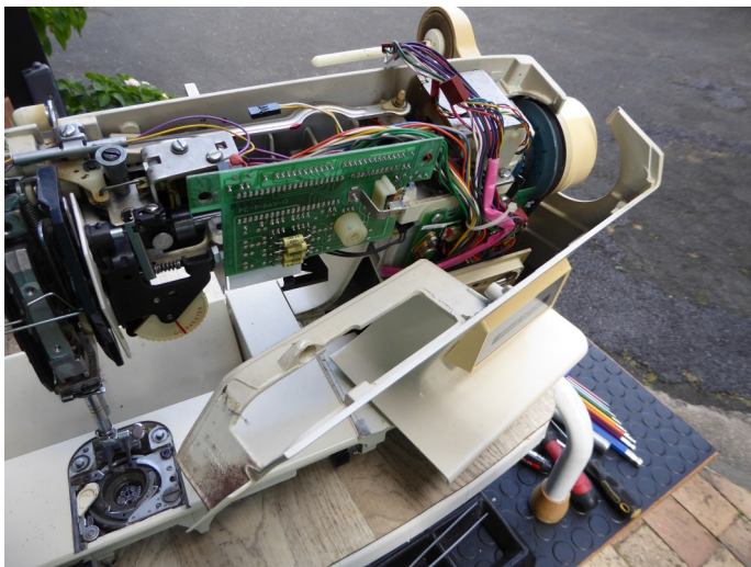
Vorderteil abnehmen
