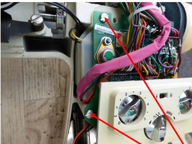
Schrauben entfernen
