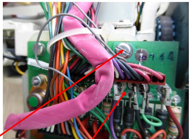
Schrauben entfernen
