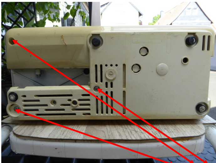
Schrauben entfernen
