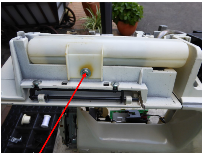
Schraube entfernen
