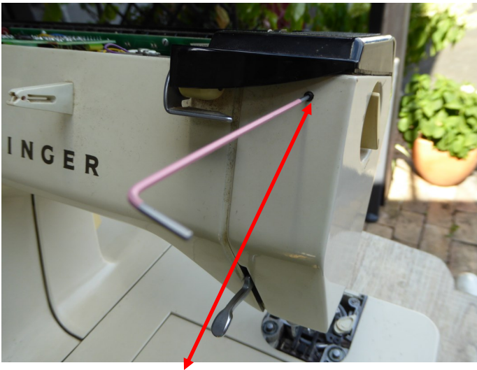
Madenschraube lösen,
